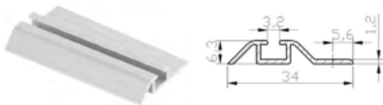
Направляющий профиль для распашной двери
